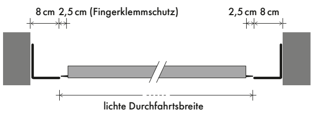
EINBAU ZWISCHEN DER LAIBUNG
