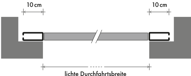
EINBAU HINTER DER LAIBUNG
