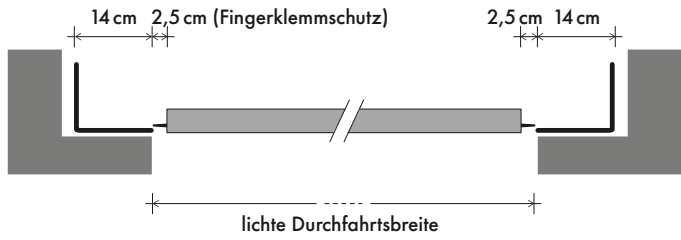
EINBAU HINTER DER LAIBUNG
