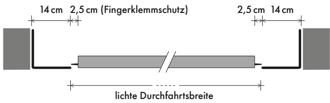
EINBAU ZWISCHEN DER LAIBUNG
