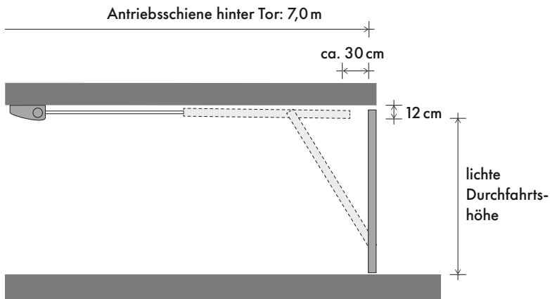
EINBAU UNTER GLATTER DECKE
